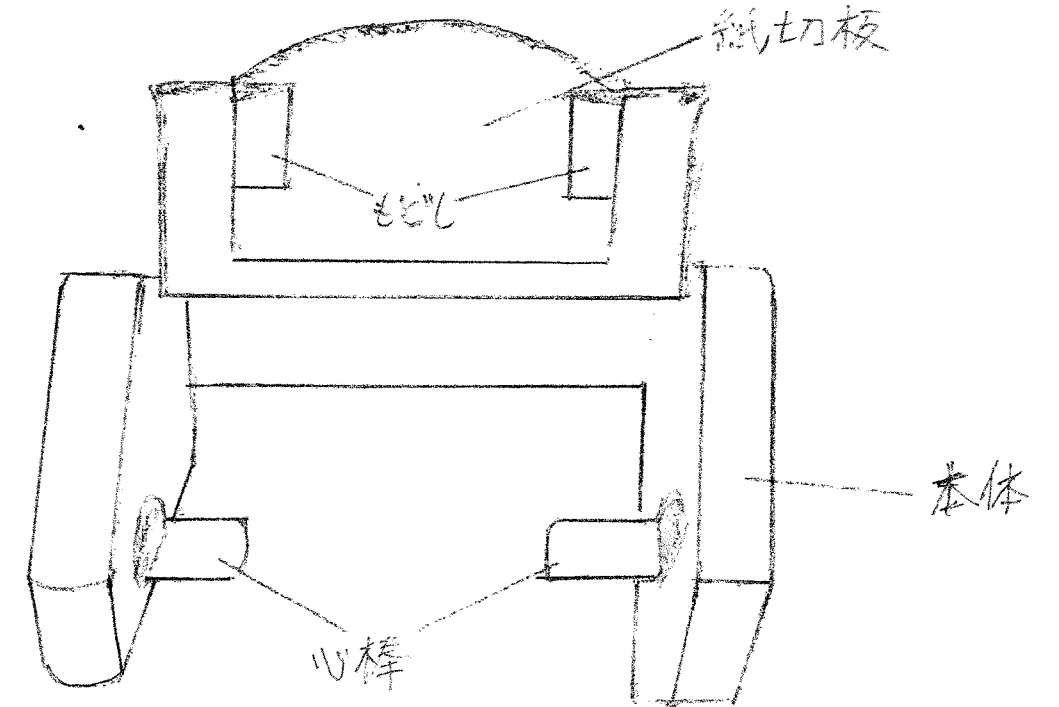
【図2】 紙切板部分
